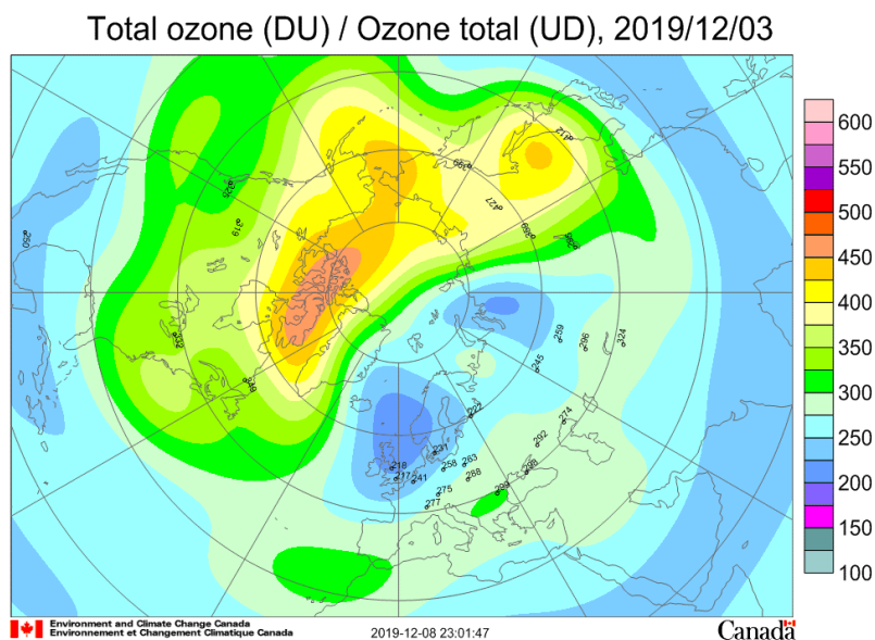
Рис. 2.13. Поле ОСО над Северным полушарием 03.12.2019 г. по данным канадского центра по окружающей среде и изменениям климата https://exp-studies.tor.ec.gc.ca . В цветовой шкале представлены спутниковые данные. В виде цифр приведены значения, полученные наземной аппаратурой
