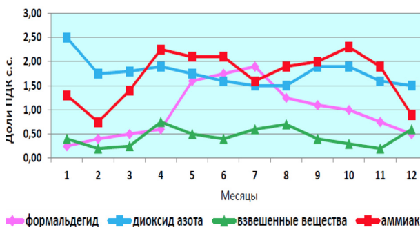
Рис. 4.3. Годовой ход концентраций взвешенных веществ, формальдегида и диоксида азота в атмосферном воздухе г. Москвы в 2019 г.
