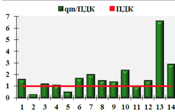
Рис. 3.18. Средние из максимальных концентрации примесей в городах России 1 – взвешенные вещества, 2 – диоксид серы, 3 – оксид углерода, 4 – диоксид азота, 5 – оксид азота, 6 – сероводород, 7 – сероуглерод, 8 – фенол, 9 – фторид водорода, 10 – хлорид водорода, 11 – аммиак, 12 – формальдегид, 13 – бенз(а)пирен, 14 – этилбензол
